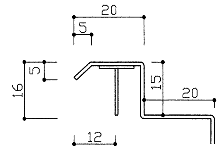
ツバ折込み詳細図
