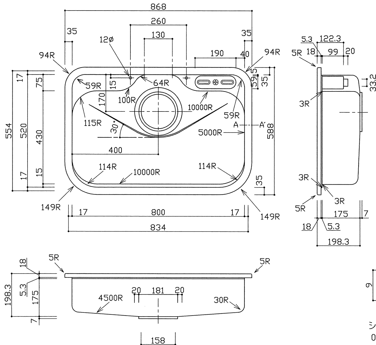
A-A' 断面詳細図
