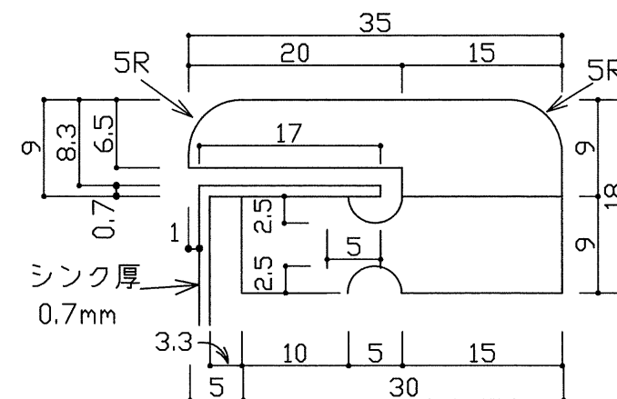
A-A' 断面詳細図
