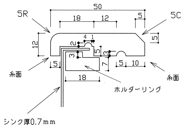
A-A' 断面詳細図
