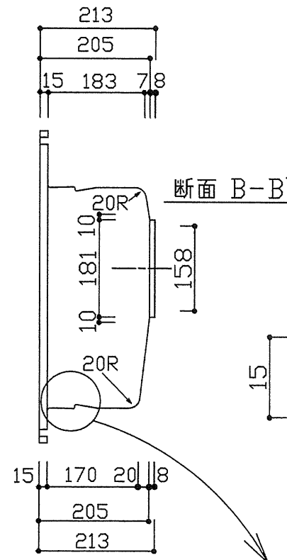
段・デッキ部 詳細図
