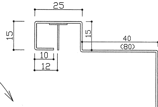
リブ部 詳細図(1/1)
