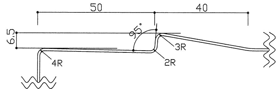
リブ部 詳細図(1/1)
